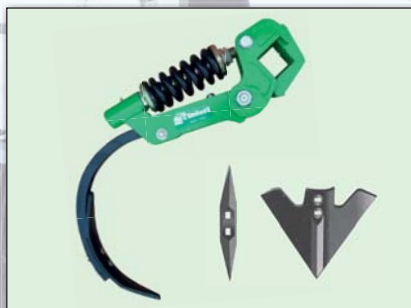
Supporto con molla doppia e braccio mm 30x30 Tine support with double spring Support du bras avec double ressort Lager mit doppelter Feder und Arm 30x30 mm. Soporte de brazo con doble muelle
